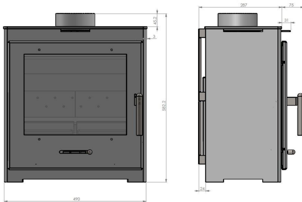
Technický výkres hede 1:
