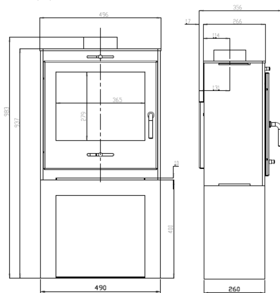
Technický výkres hede 1D:
